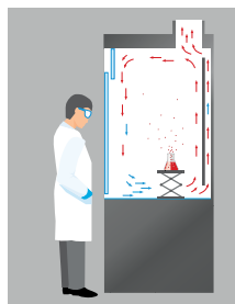
Abbildung 21: Geschlossener Frontschieber, Normalbetrieb.
