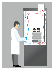
Abbildung 22: Vermeidung der Störung der Luftwalzen durch „Sperreige Aufbauten“.
